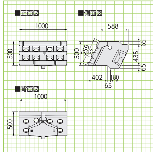
D型 参考重量:221kg 胴込量:0.228m 3
