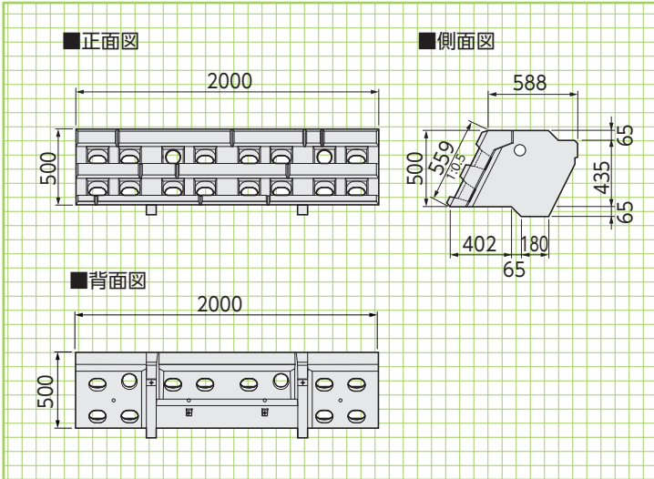
C型 参考重量:411kg 胴込量:0.472m 3
