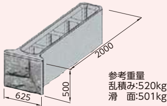
③ 製品吊り降ろし
