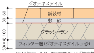
■表 1:歩行者系道路の舗装構造例 【標準品, リサイクル, 保水】
