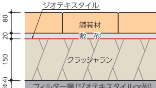
■表 5:歩行者系道路の車両乗入れ部の舗装構造例
