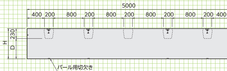
■正面図
