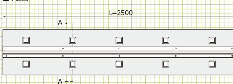
■平面図
