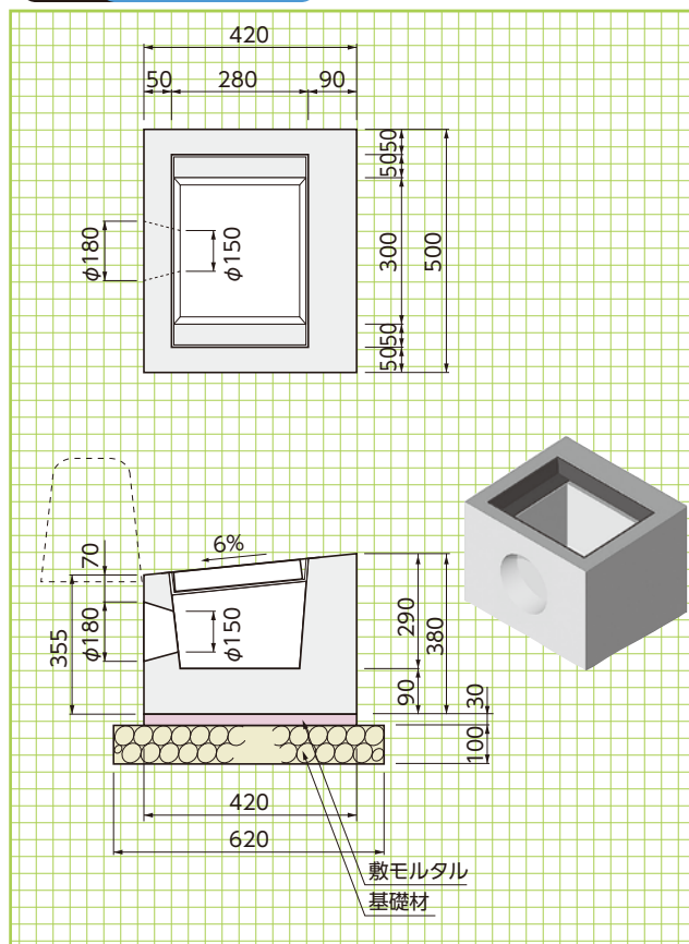
II型 製品重量=116kg
