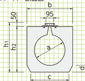
■A-A' 断面図
