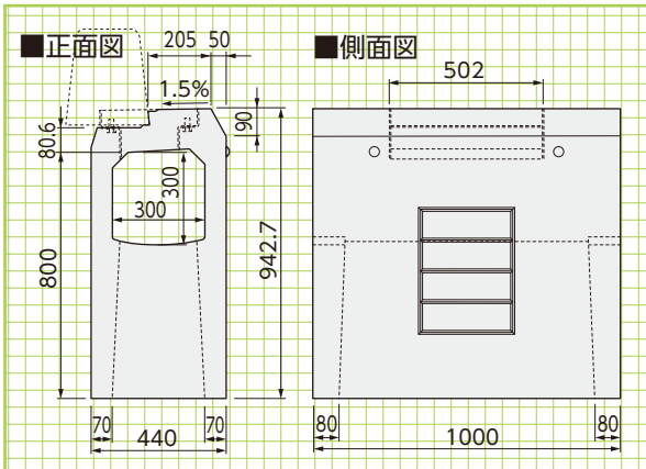
400×400用専用柵
