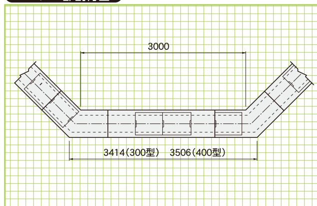
コーナ一部割付図
