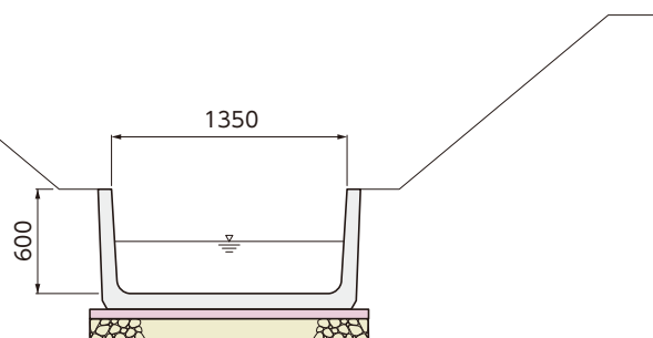
■左写真参考断面図
