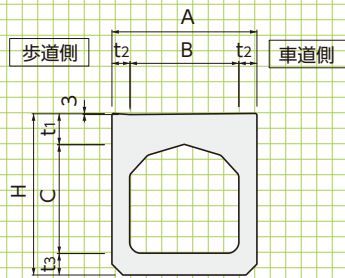
■A-A断面図
