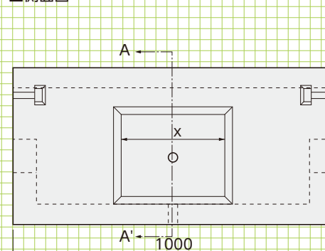
■平面図
