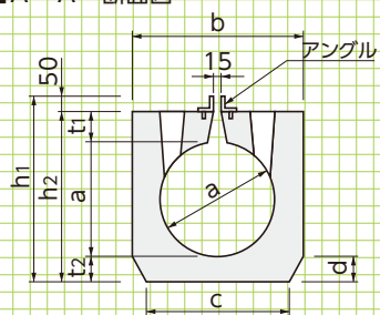
■A-A' 断面図
