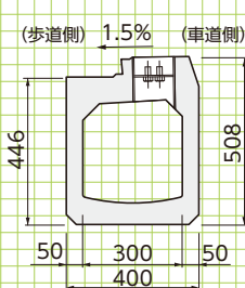
■A-A'断面図
