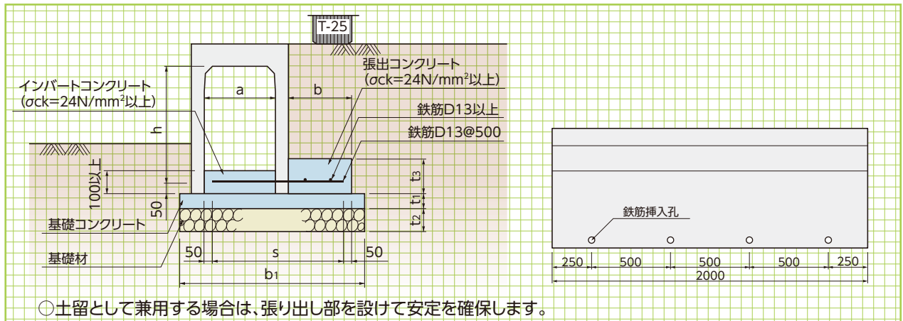
■張り出し部の寸法表
