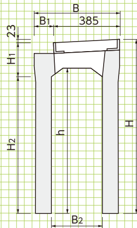
■断面図
