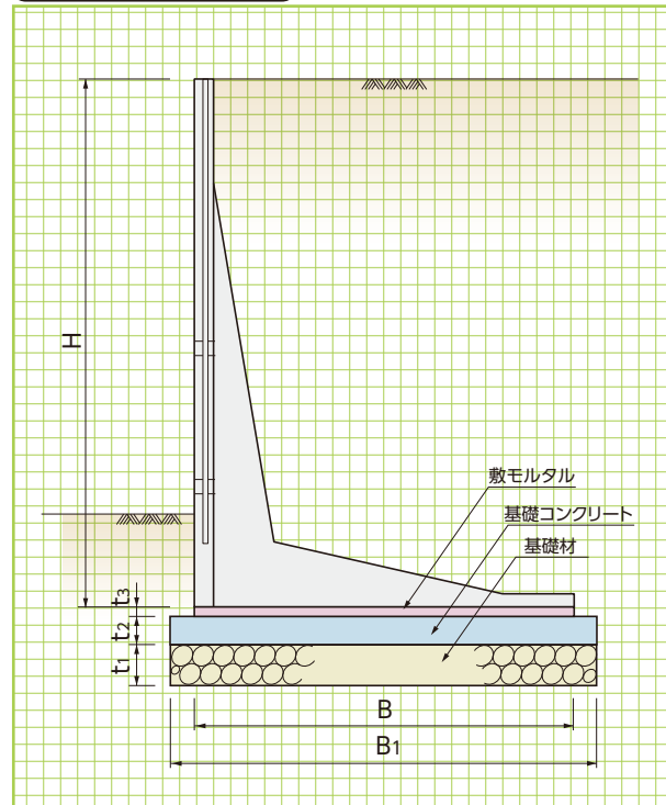
標準敷設図
