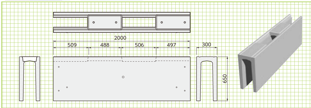
形状・寸法
