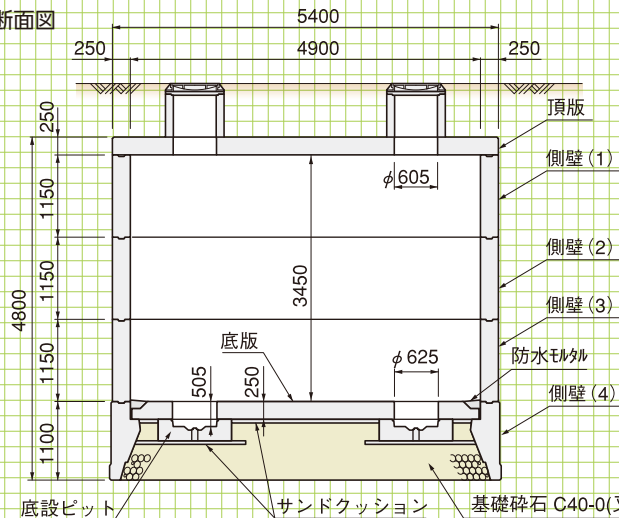
■B-B断面図
