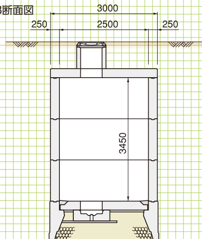
■B-B断面図
