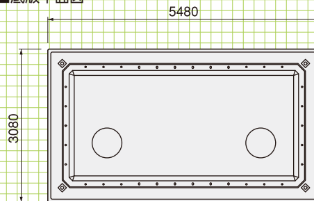
■底版平面図
