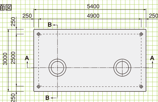
底板組立
