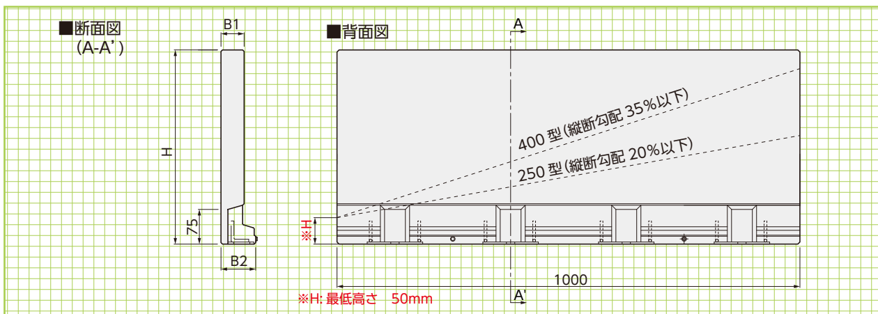
基本形状図
