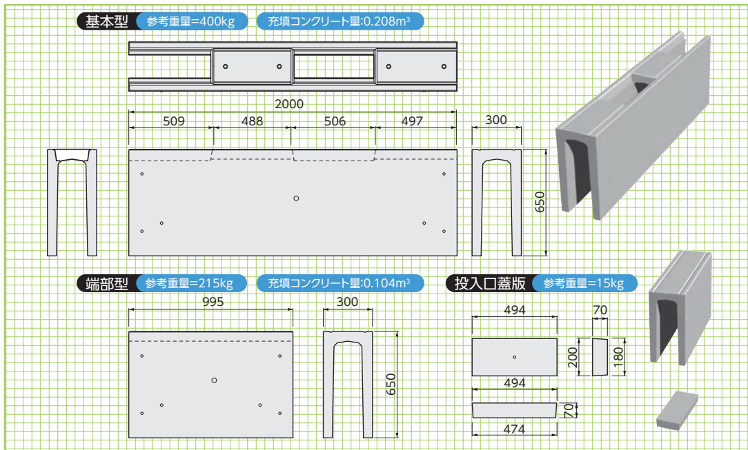
基本形状図
