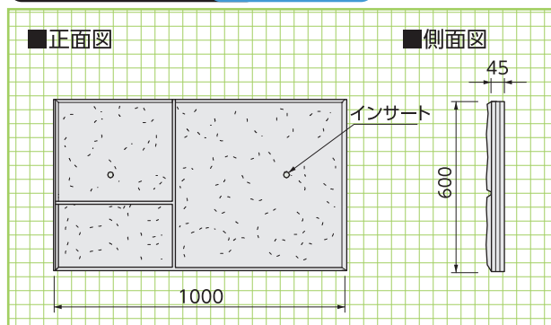
底版ブロック 参考重量=43kg
