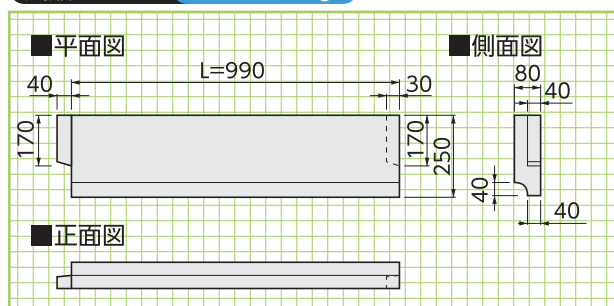
底版ブロック 参考重量=43kg
