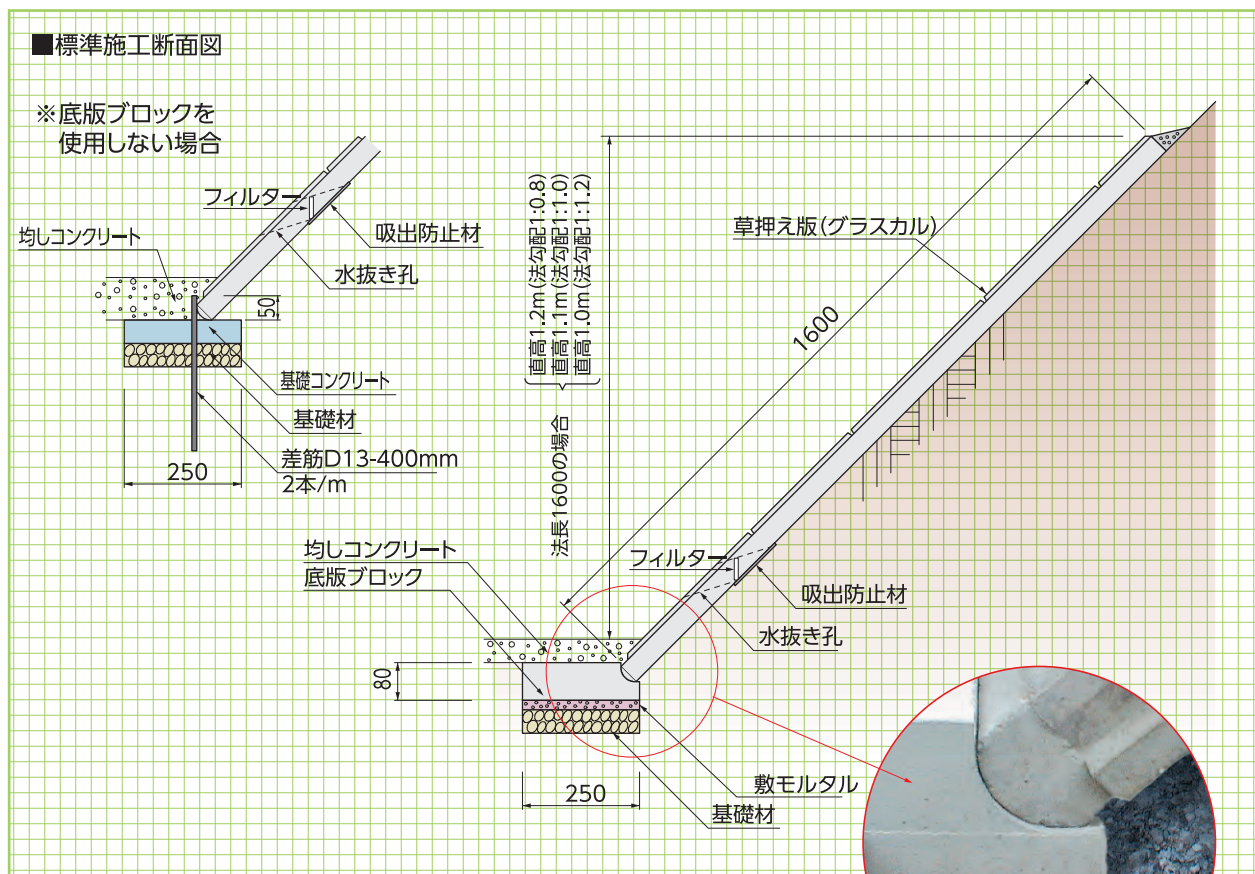
標準施工断面図
