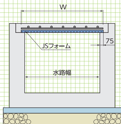
■打設断面図
