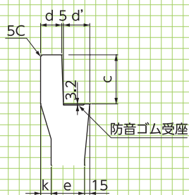
■蓋掛け部 詳細図
