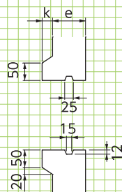
■目地部 詳細図
