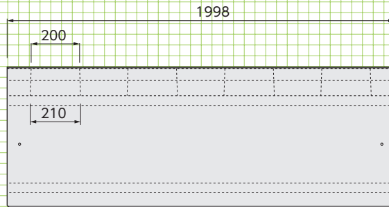
■側面図
