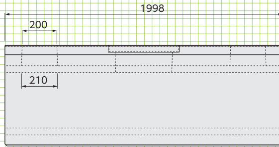
■側面図
