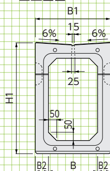
■正面図
