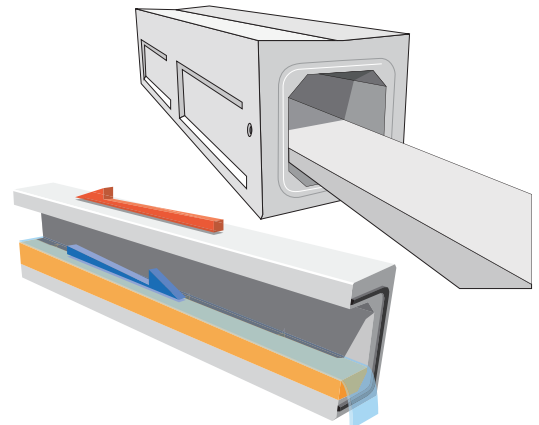
プレキャストインバートブロック
