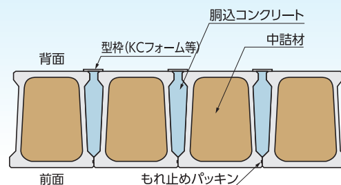
■敷設平面図
