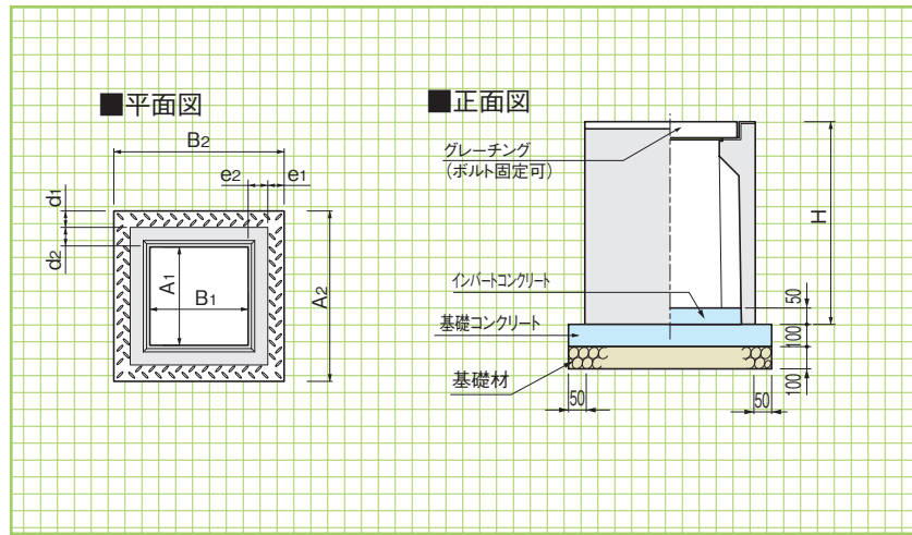
基本形状図
