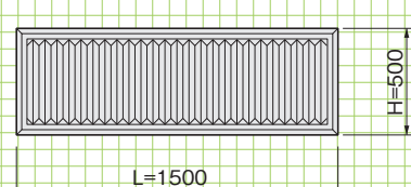
■正面図
