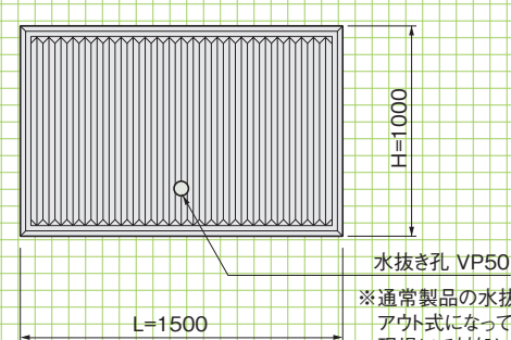
■側面図
