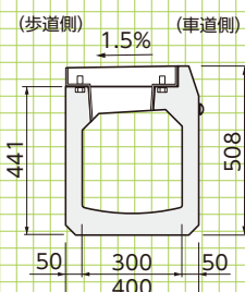
■A-A'断面図
