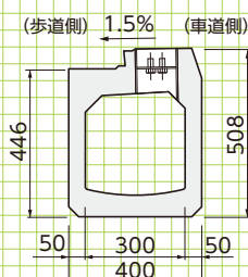
■A-A'断面図
