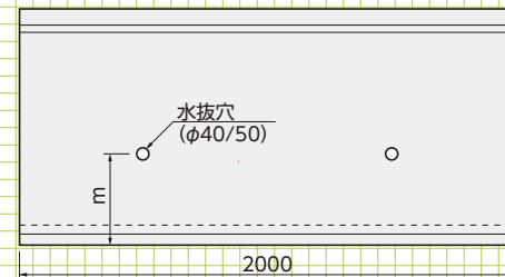
■正面図
