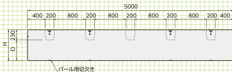
■正面図
