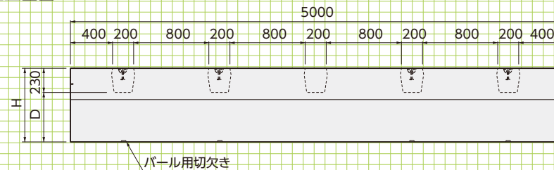
■正面図
