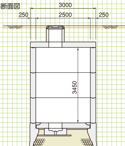
■B-B断面図
