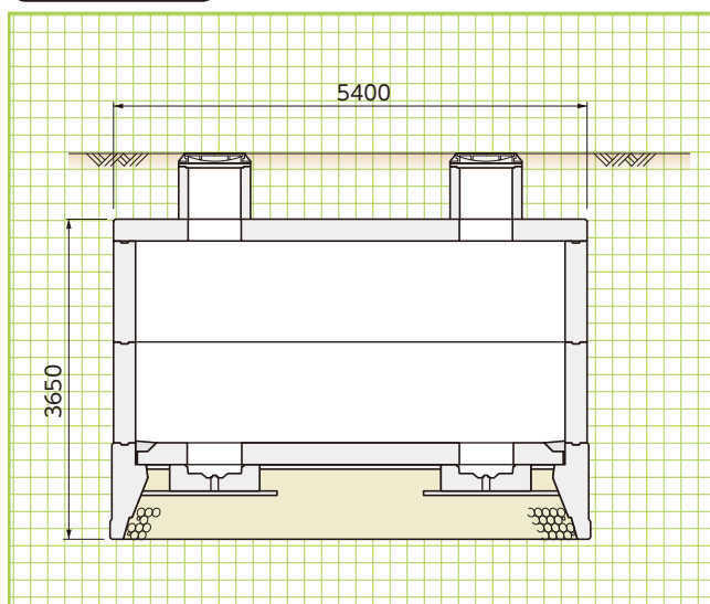
〈縦置き25型〉
