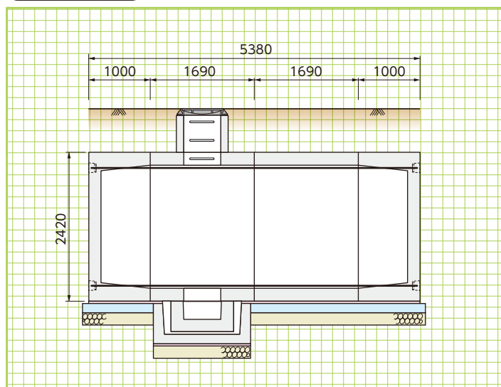
〈横置き29型〉
