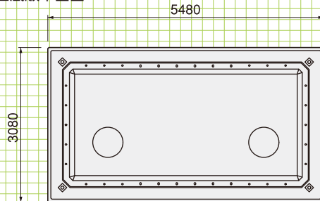
■底版平面図
