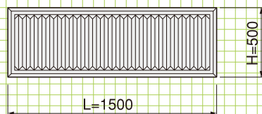
■正面図
