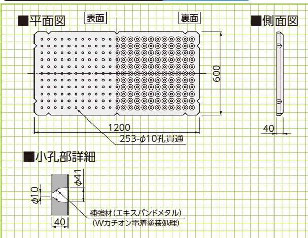
基本形状図
