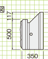
■側面図
