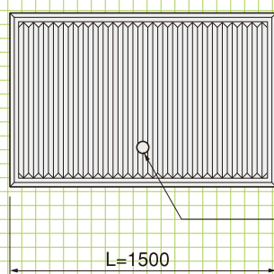
■正面図
