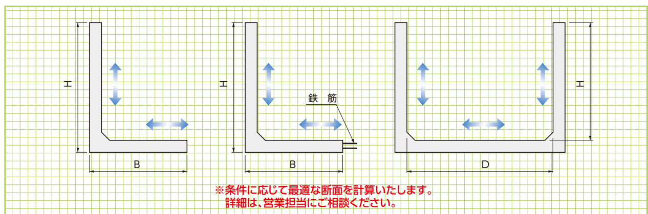
基本形状図
