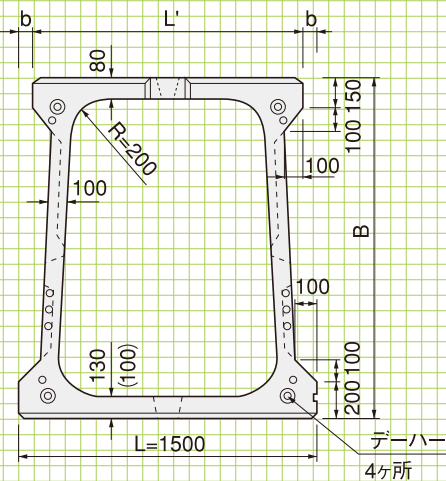
■平面図
