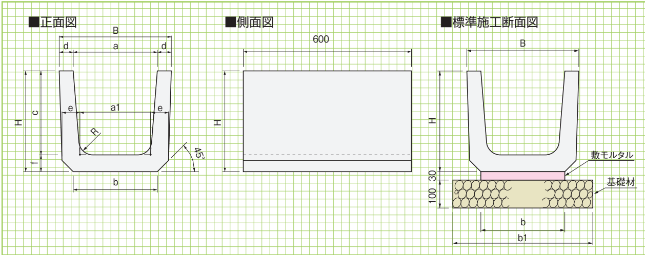
基本形状図
