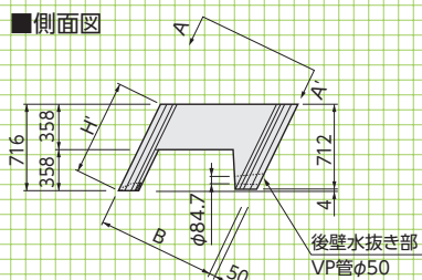
■側面図
