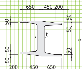
■A-A'断面図
