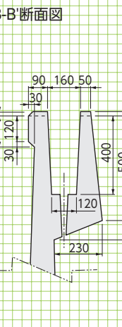
■B-B'断面図
