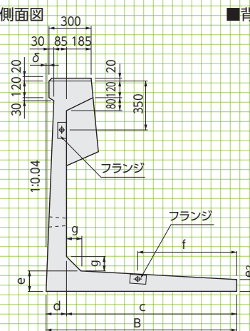
■側面図
