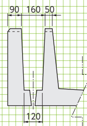
■A-A断面図
