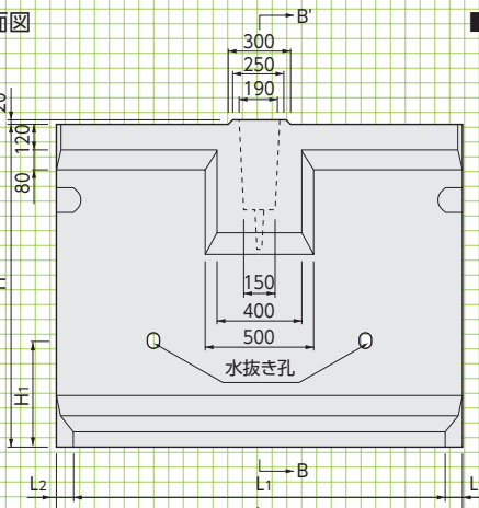
■背面図
