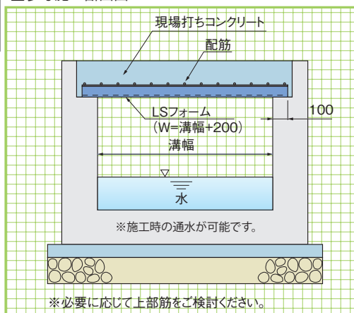
施工断面図 製品構造図
