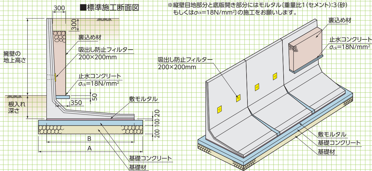
■コンクリート基礎工による標準敷設材料表
