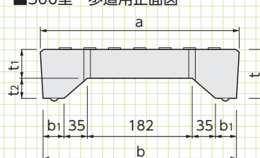
■300型 歩道用正面図
