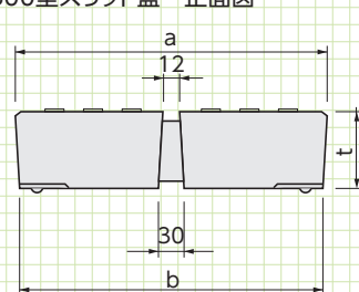
■300型スリット蓋 正面図
