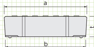
■300型 歩道用正面図
