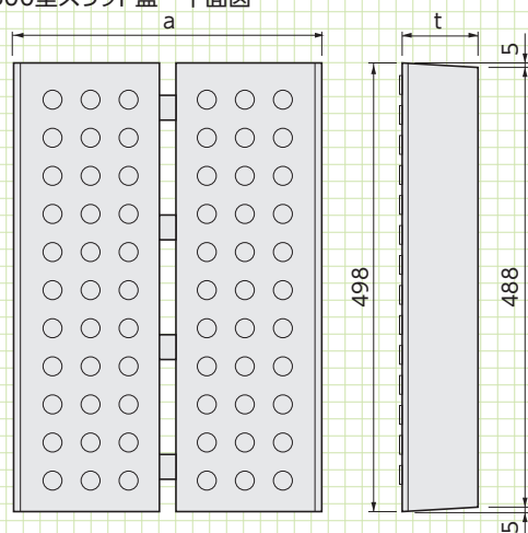
■300型スリット蓋 平面図
