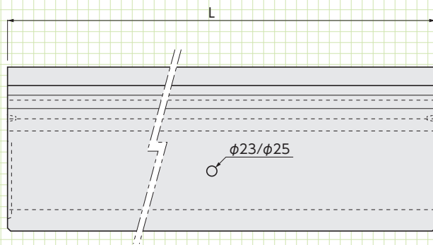
■側面図
