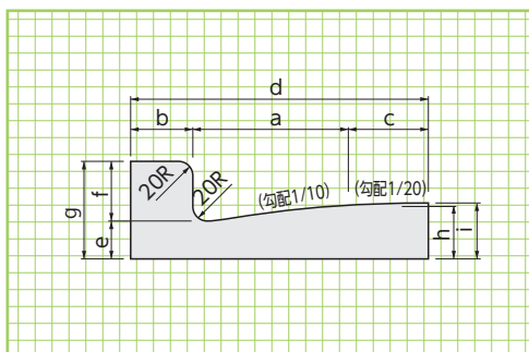
基本形状図
