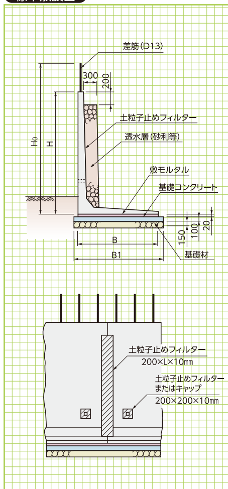
標準敷設図
