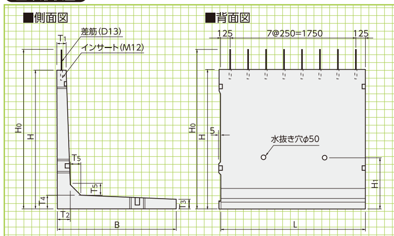
基本形状図
