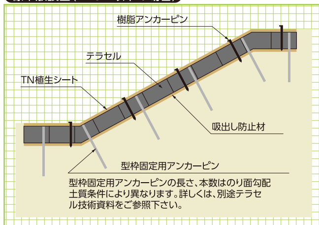
標準敷設図(H=5m以下の場合)
