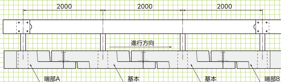
■接続詳細図
