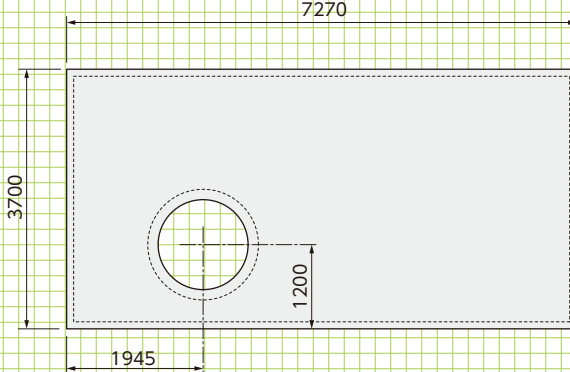
■基礎コンクリート平面図 (ピット部用基礎使用)
