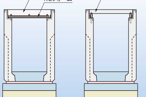
▼施工後
