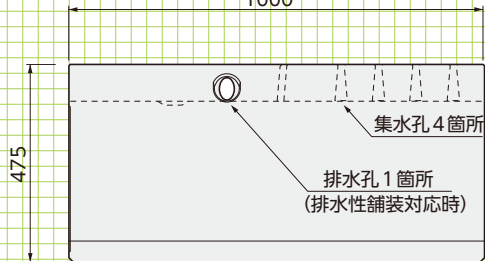
■側面図
