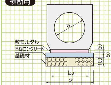
■横断用
