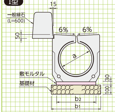
■横断用
