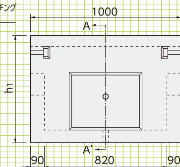
■側面図
