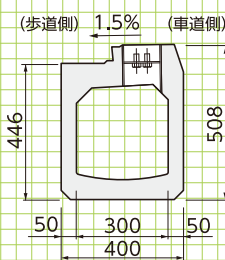
■A-A'断面図
