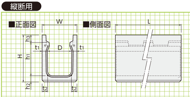
■寸法・重量表(縦断用) ※ ( )内の数字はL=2000の重量です。
