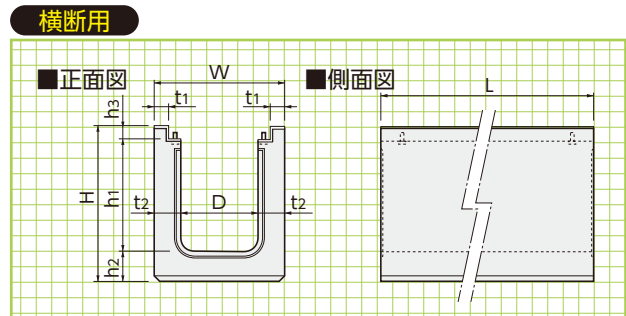
■寸法・重量表(横断用) ※ ( )内の数字はL=2000の重量です。
