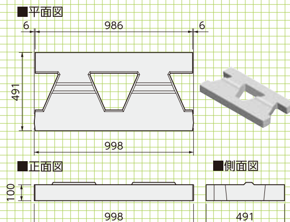
基礎ブロック 参考重量:87kg
