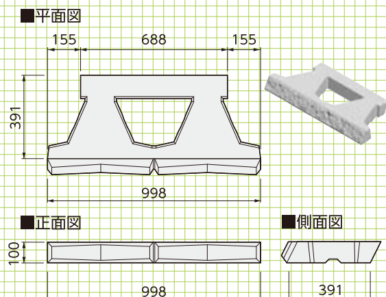
天端ブロック 参考重量:58kg
