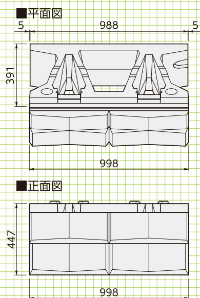
I 型 参考重量:225kg
