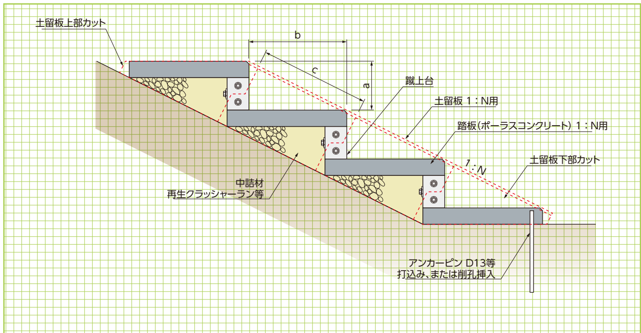
標準構造図
