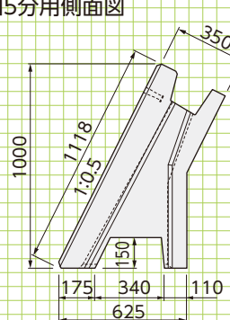
■5分用側面図
