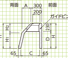
■断面図
