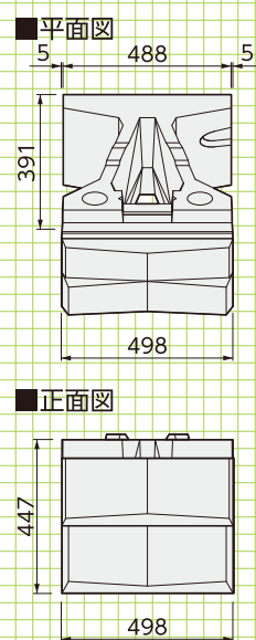
II 型 参考重量:112kg
