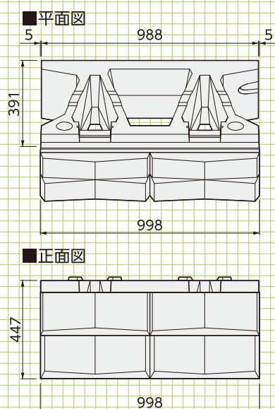
天端ブロック 参考重量:58kg
