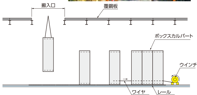
■断面図
