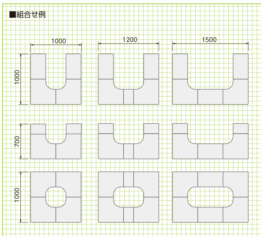
基本形状図
