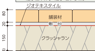
■表 5:歩行者系道路の車両乗り入れ部の舗装構造例
