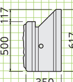
■側面図
