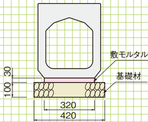
■標準敷設図
