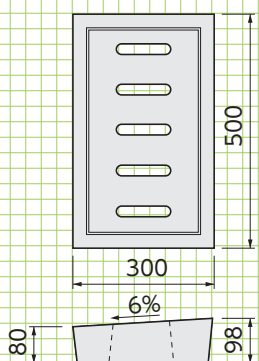
■平面図
