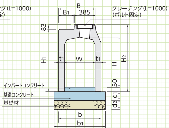
■断面図 (W=500,600)
