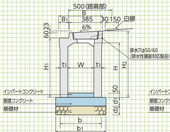
■断面図 (W=300,400)
