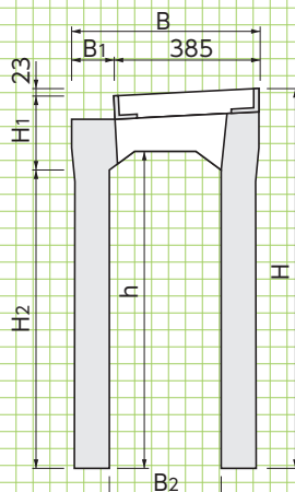
■断面図
