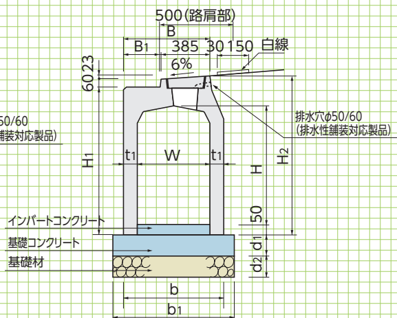
■断面図 (W=500,600)
